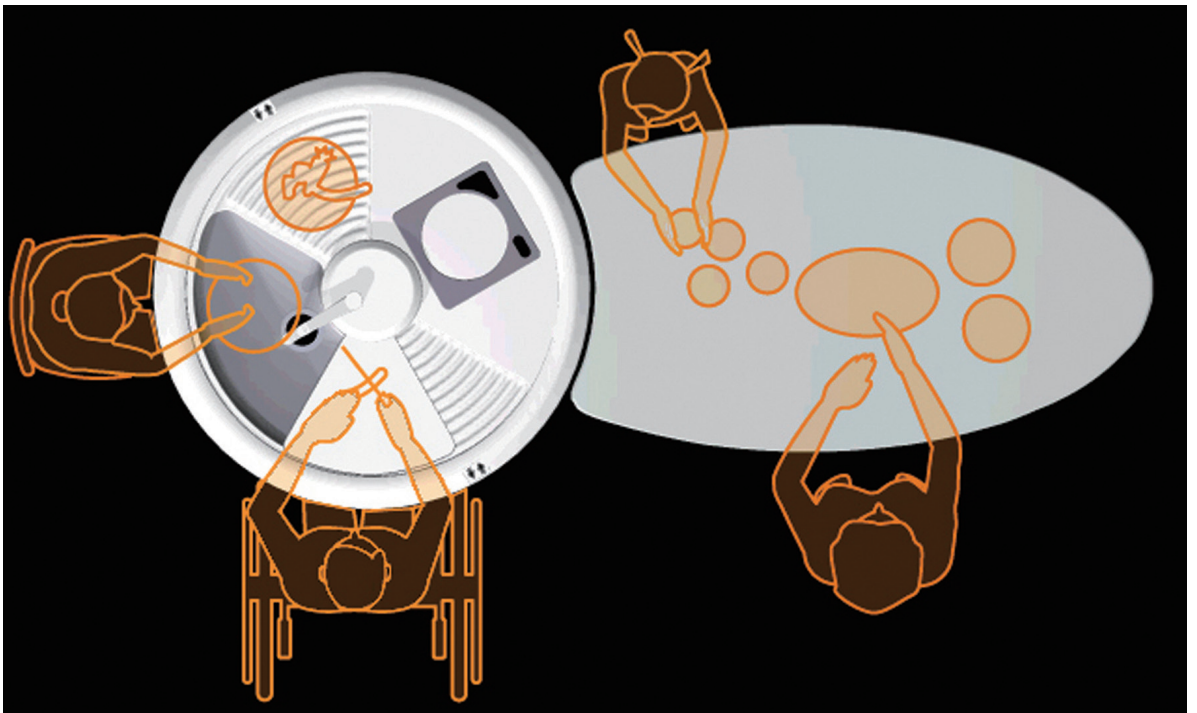
「バリアフリー・キッチン」INAX・大林組・イトーキ, 1997 / 椅座位や車いすでも使用できるキッチン シンク、コンロ、調理台を円形に配置し、回転させることで横移動せずに作業できる / 身長、姿勢あるいは作業内容に応じて高さを容易に変えられる
