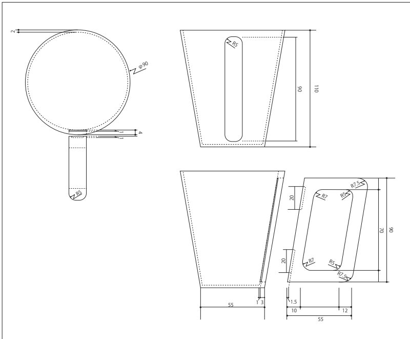
図1: 寸法図
